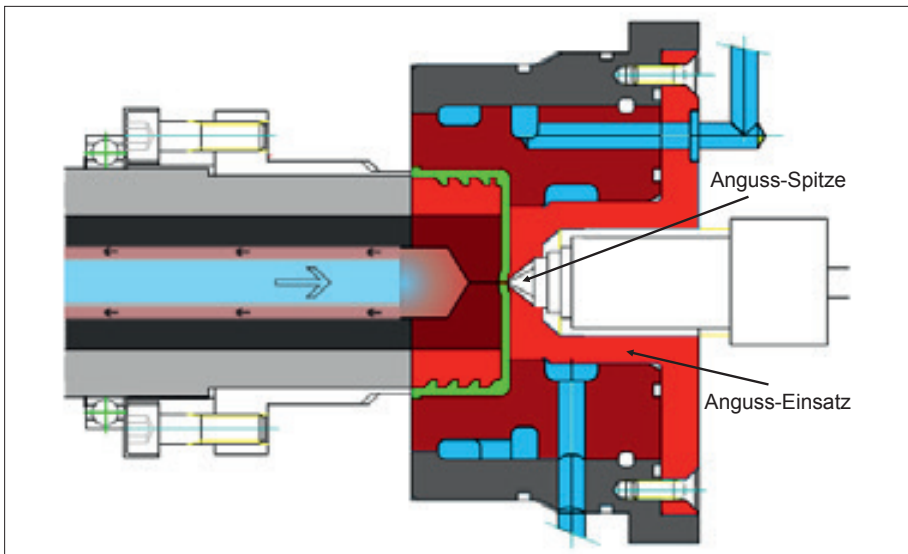
Bild 3: Schematische Darstellung der Positionierung der Anguss-Spitze.
